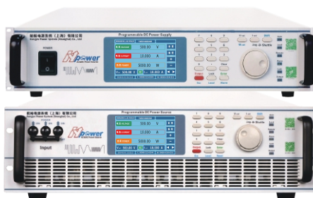
19英寸2U@5kW
